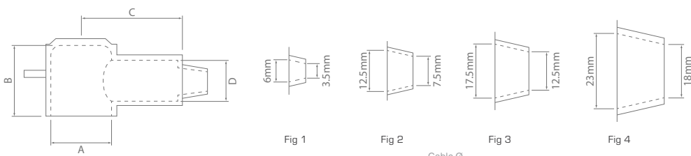
Cable Ø
